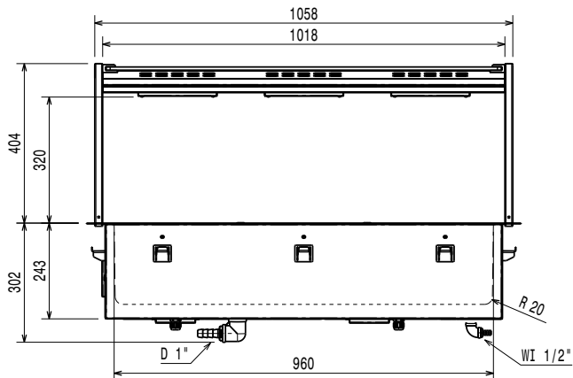
Front aanzicht
